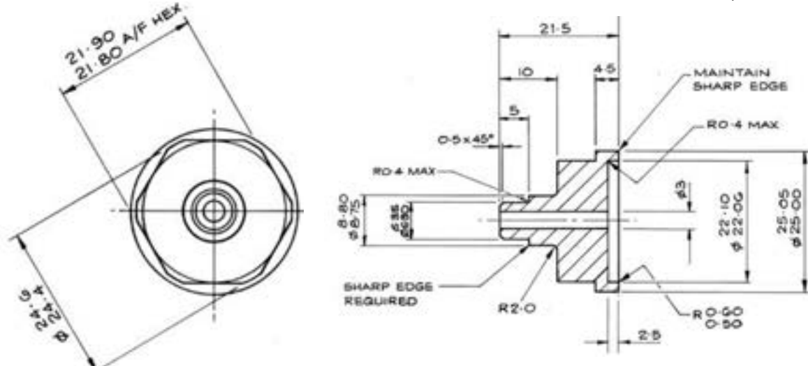
227-270 Conn VCR Vacuseal Adapter D25 A-A3-1886$2
