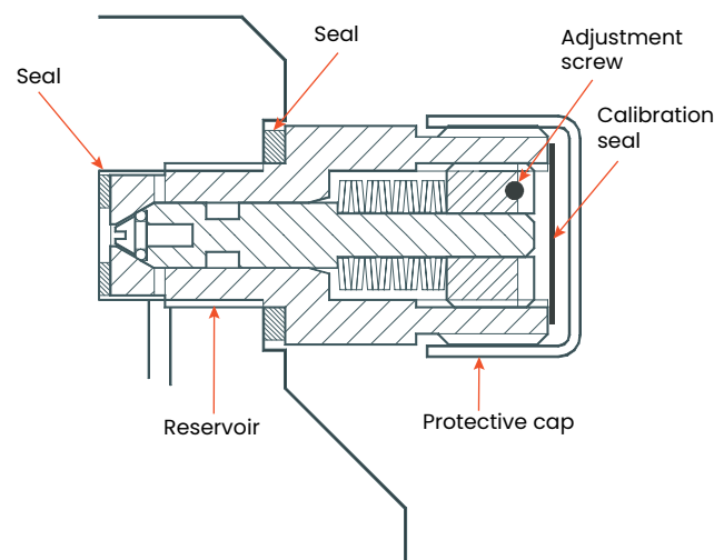
PRV212 schematic
